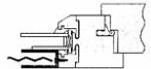
Montage der Seitenführung bei FL Montage:
