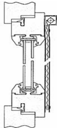
Montage der Seitenführung bei FL Montage:
